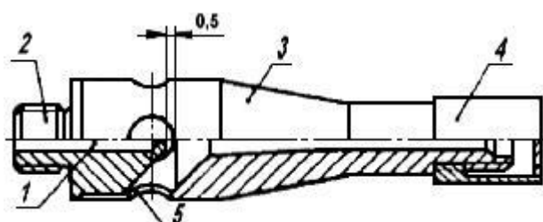
Рисунок Е.1 - Общий вид газовой горелки
