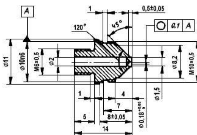
Рисунок Е.2 - Газовое сопло горелки
